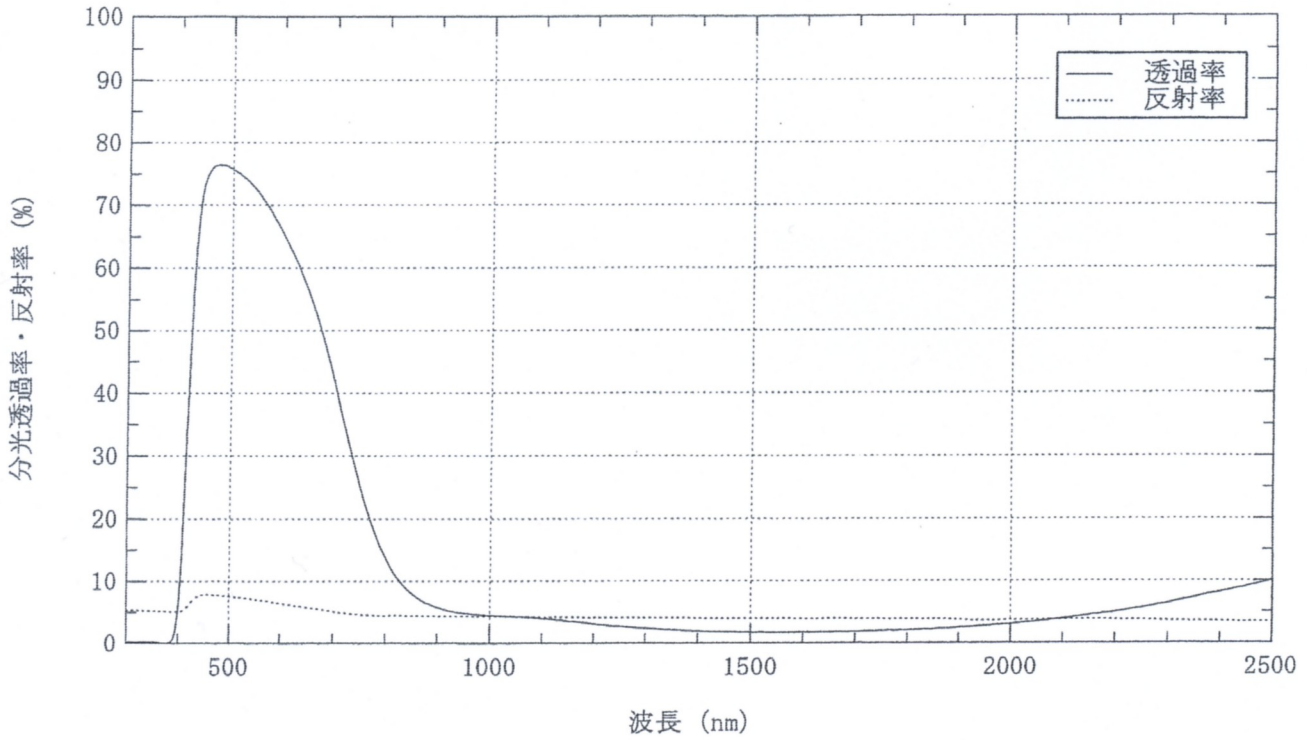
図-1 分光透過率, 反射率測定結果 (300~2500nm)
